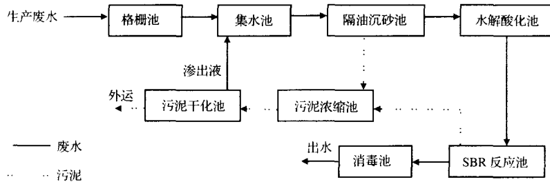
图 1 废水处理工艺流程图
