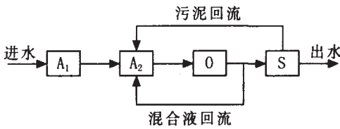
A 1 —厌氧池(酸化水解池) A 2 —缺氧池 O—好氧池 S—沉淀池
